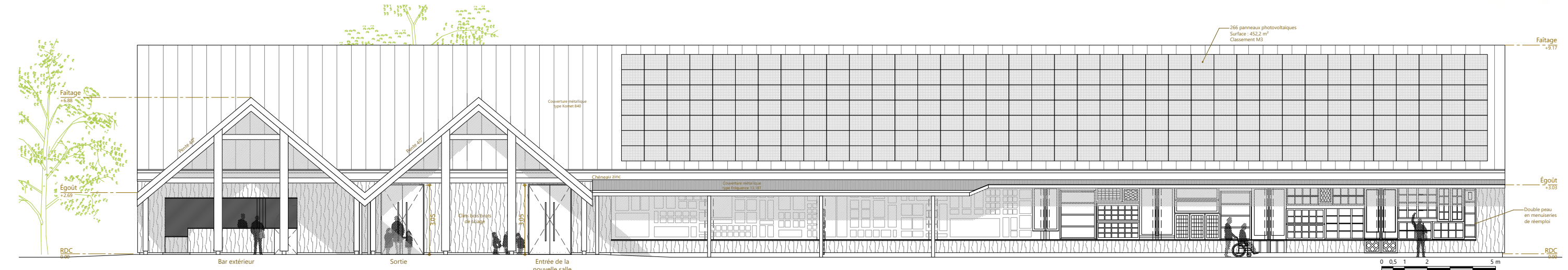
Élévation Sud-Ouest
