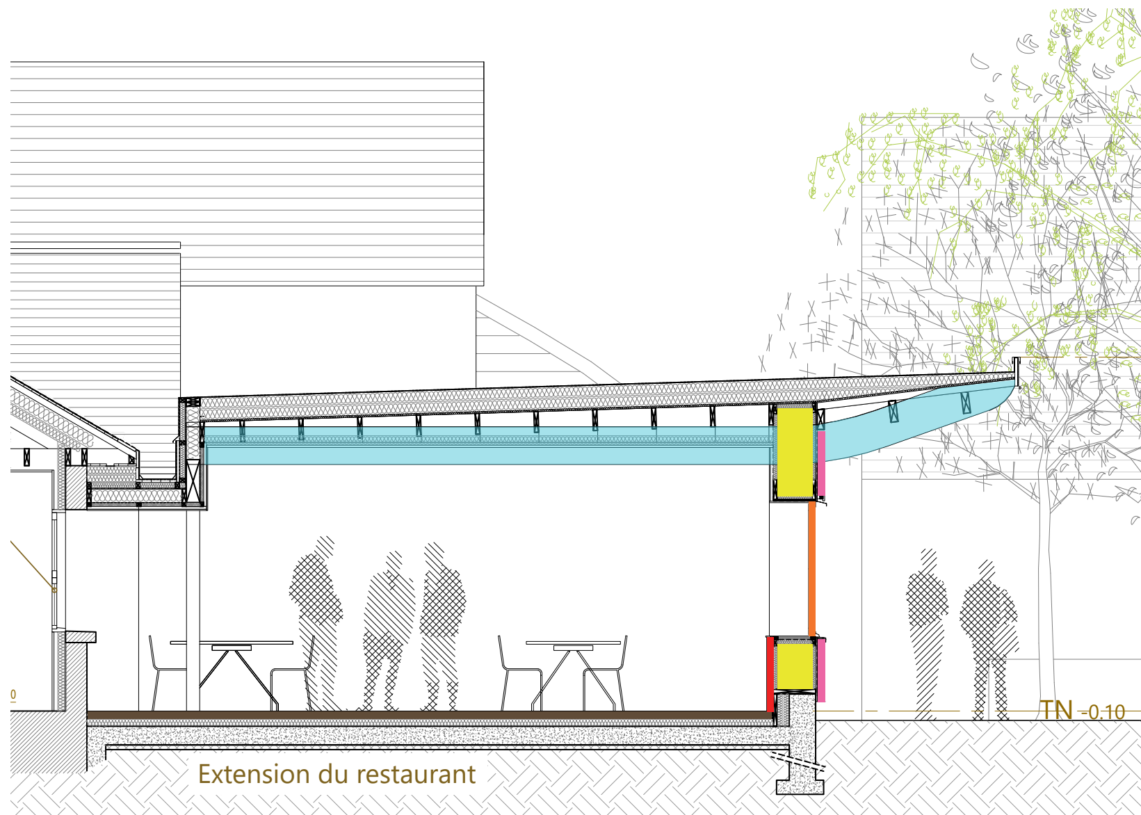
Coupe sur la grande salle
