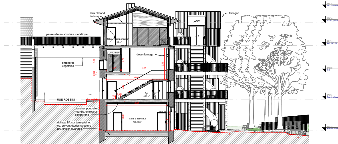
Coupe transversale
